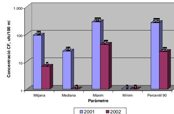
COMPARACIÓ QUALITAT AIGUA REGENERADA TERCIARI EDAR CASTELL-PLATJA D'ARO
