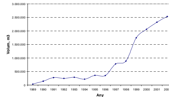
EVOLUCIÓ DE LA PRODUCCIÓ D'AIGUA REGENERADA EN LA COSTA BRAVA (1989-2002)
